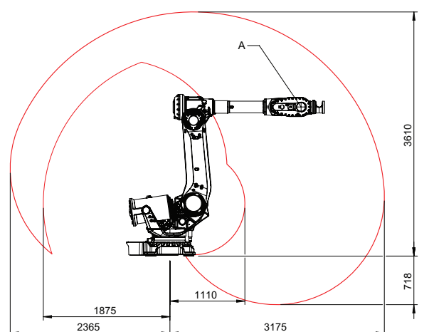
IRB 6740-220/3.2 LID 工作范围
