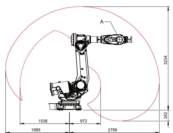
IRB 6740-270/2.8 LID 工作范围
