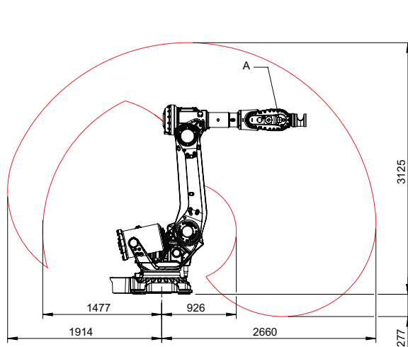
IRB 6710-175/2.65 LID 工作范围
