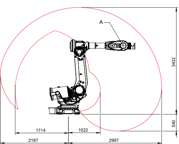
IRB 6740-230/3.0 LID 工作范围
