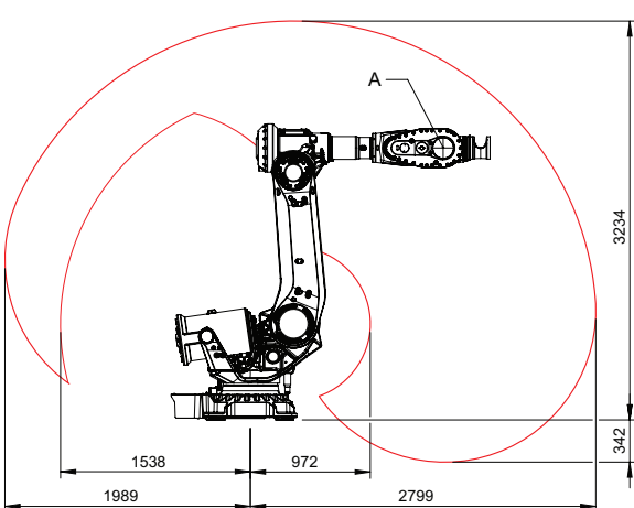
IRB 6740-270/2.8 LID 工作范围
