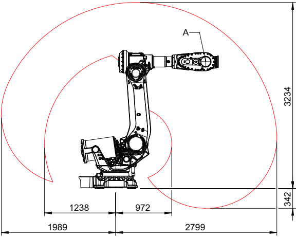
IRB 6740-310/2.8 工作范围
