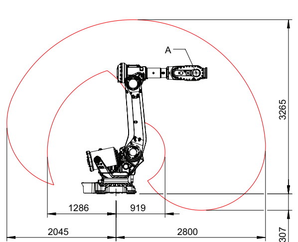
IRB 6720-210/2.8 工作范围
