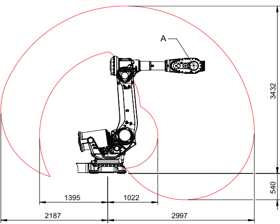
IRB 6740-260/3.0 工作范围
