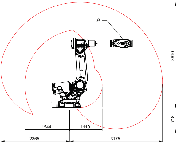
IRB 6740-240/3.2 工作范围
