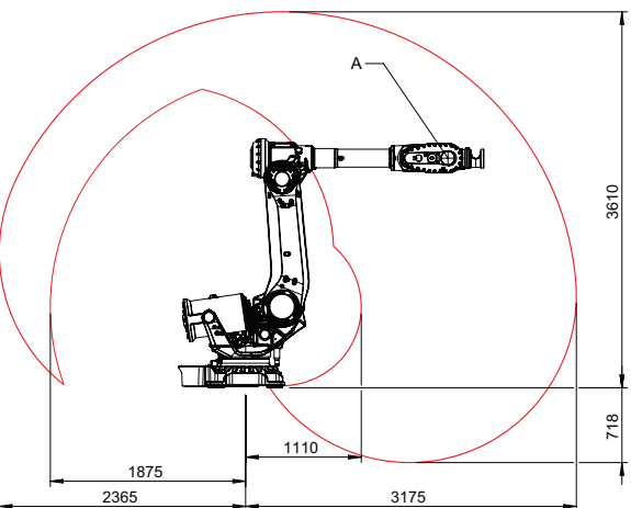
IRB 6740-220/3.2 LID 工作范围
