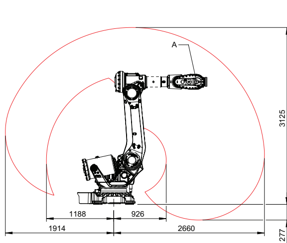
IRB 6710-210/2.65 工作范围
